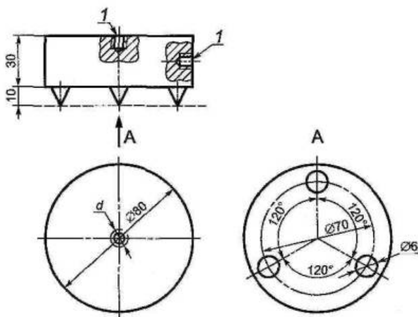
Рисунок 1 - Устройство для быстрой установки акселерометра
